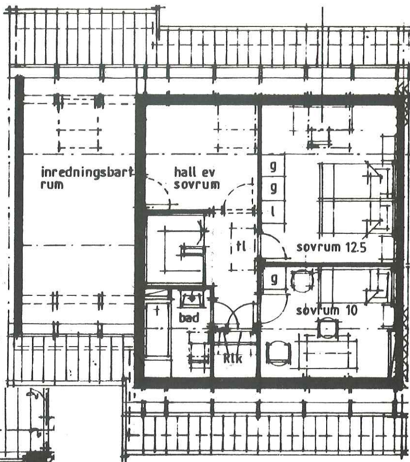
ÖVRE PLAN
