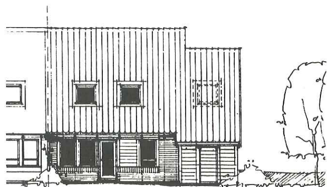
TRÄDGÅRDSFASAD
